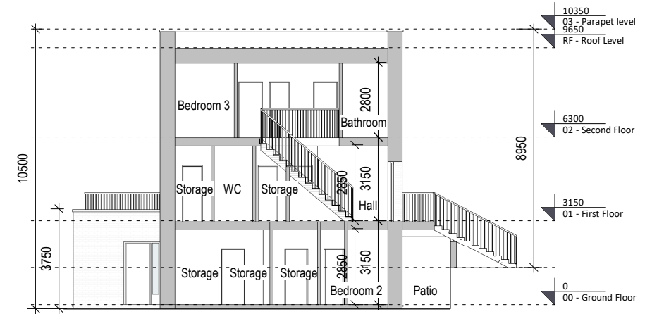
⑤ Section 1 1 : 200
