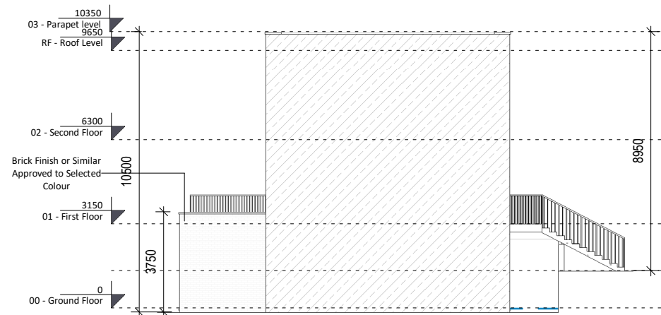
④ Right Elevation 1 : 200
